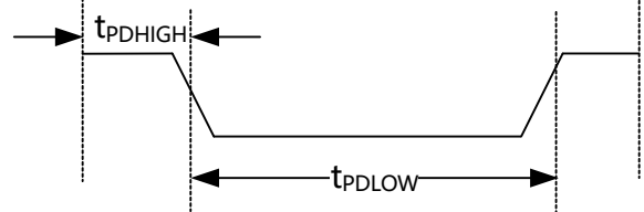
图 18 时序图
