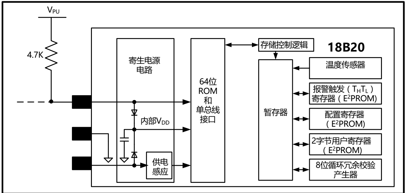
图 1 DS18B20 框图
