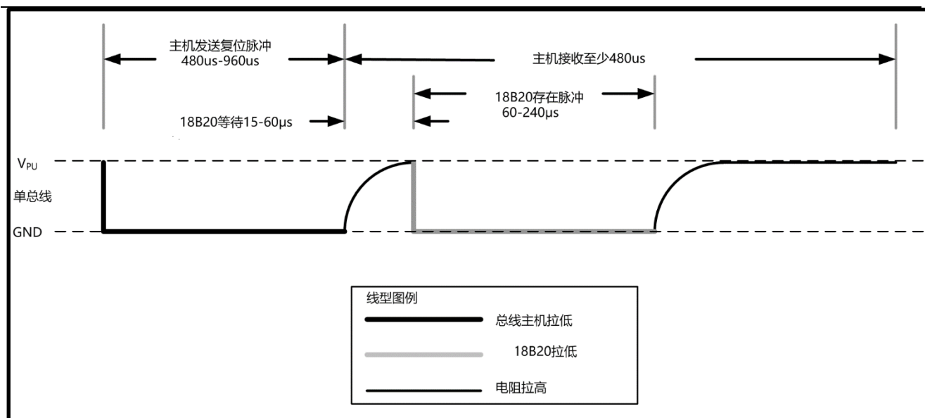
图 13 初始化时序
