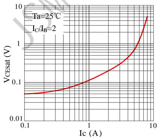
Fig5 VCESat-Ic
