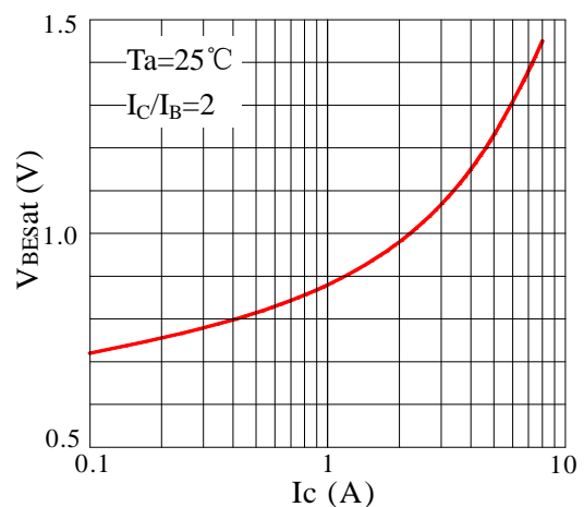
Fig6 VBESat-Ic
