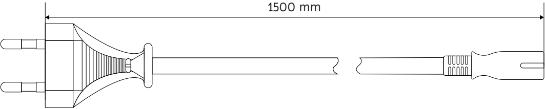
Wymiary i budowa kabla
