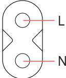
Rozkład połączeń we wtyku urządzenia
